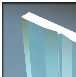
Detail Rillenschliff: doppelte Rille „Off Center“
